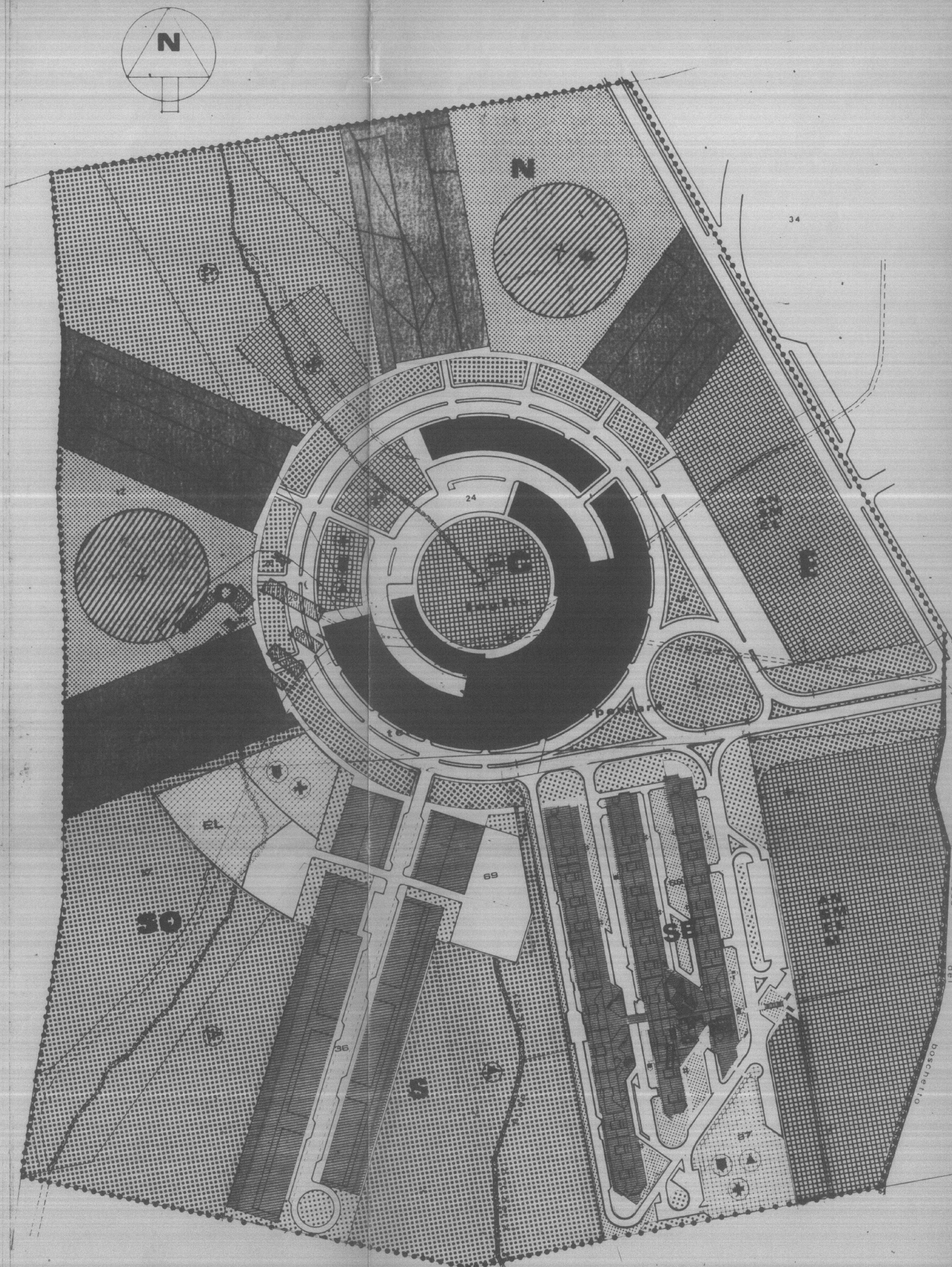
VARIANTE I.A.C.P. 12 - 1977
