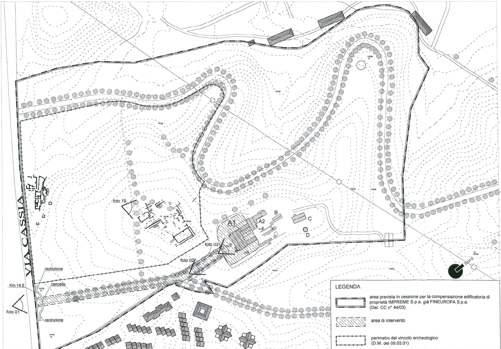
Planimetria Generale con andamento altimetrico e principali alberature esistenti (Pinus)
