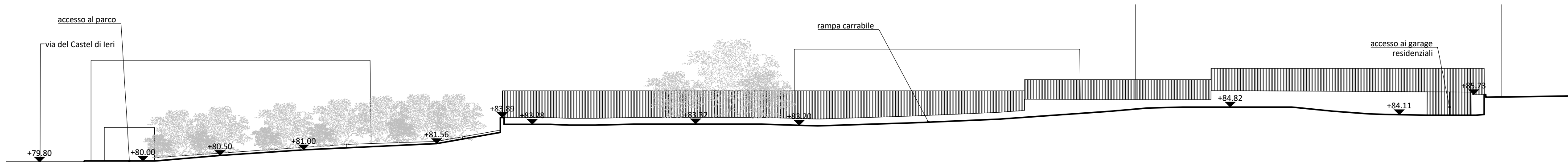
Sezione di rilievo C-C' - scala 1:300
