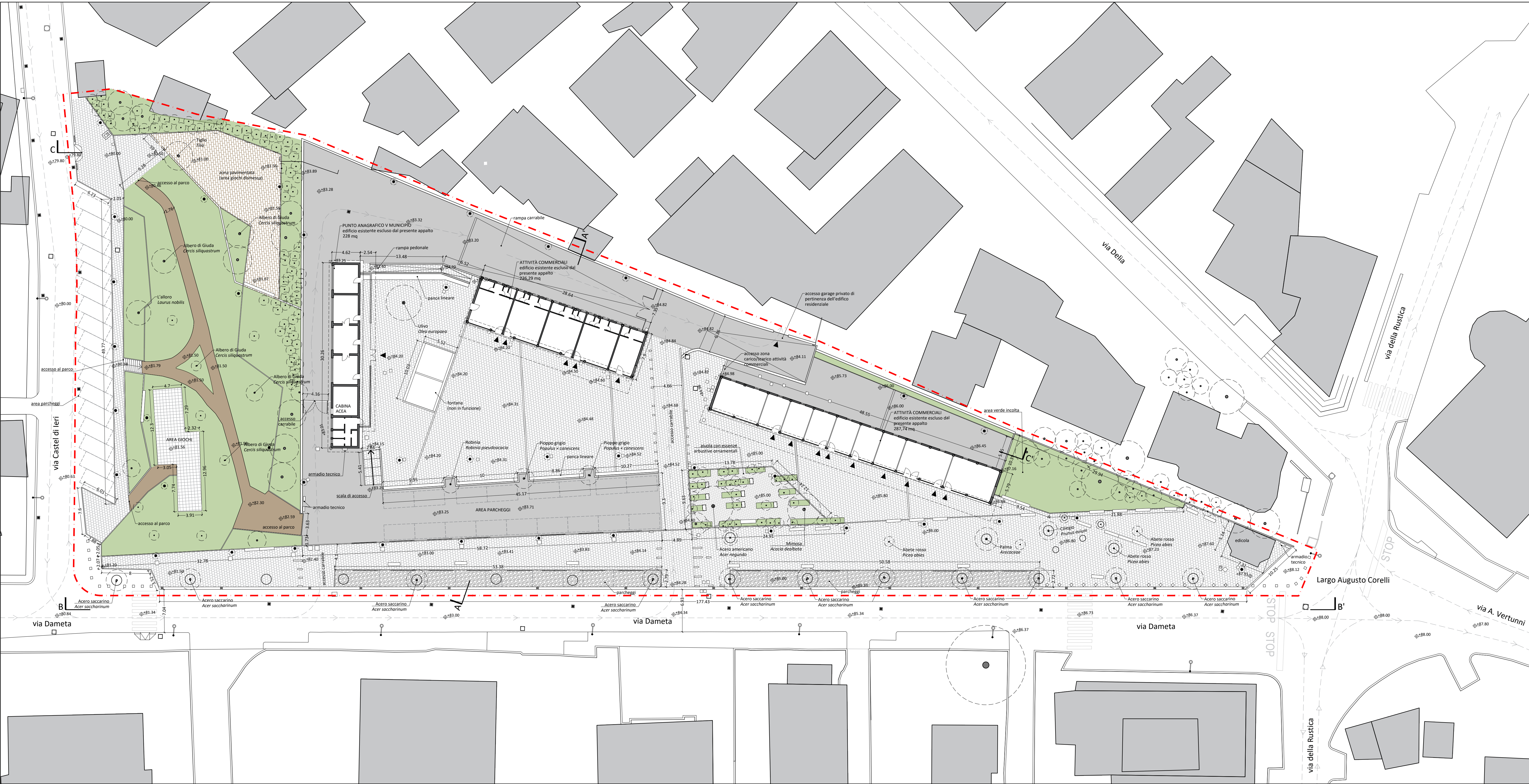
Planimetria di rilievo - scala 1:300
