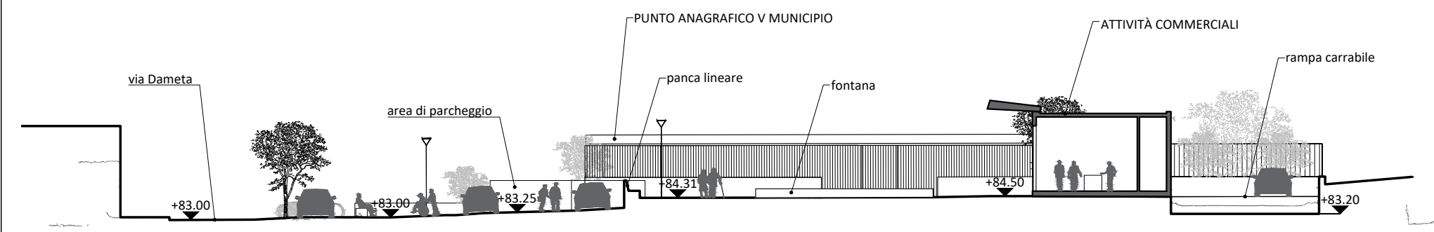
Sezione di rilievo A-A' - scala 1:300
