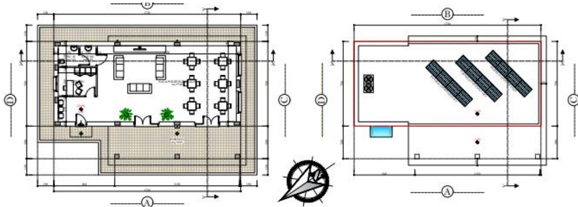
PIANTA PIANO TERRA Rapp. 1:100
