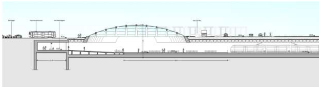
SEZIONE LONGITUDINALE
