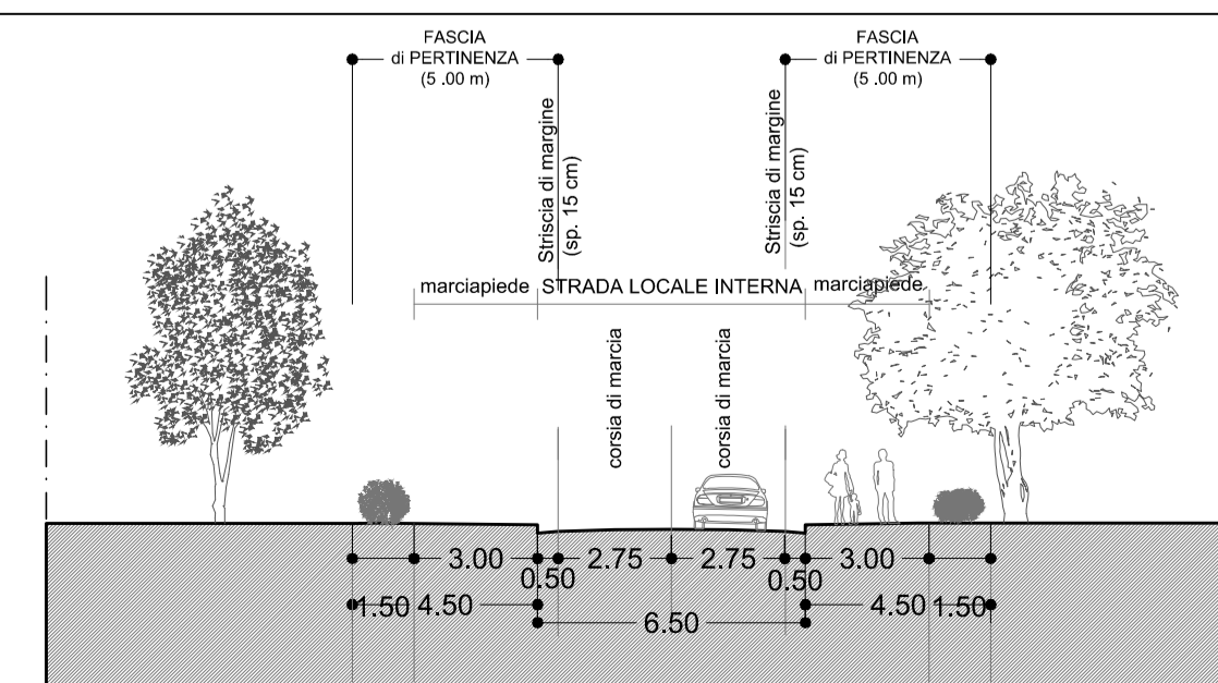
1 SEZIONE A-A': Strada Locale Interna Scala 1:200
