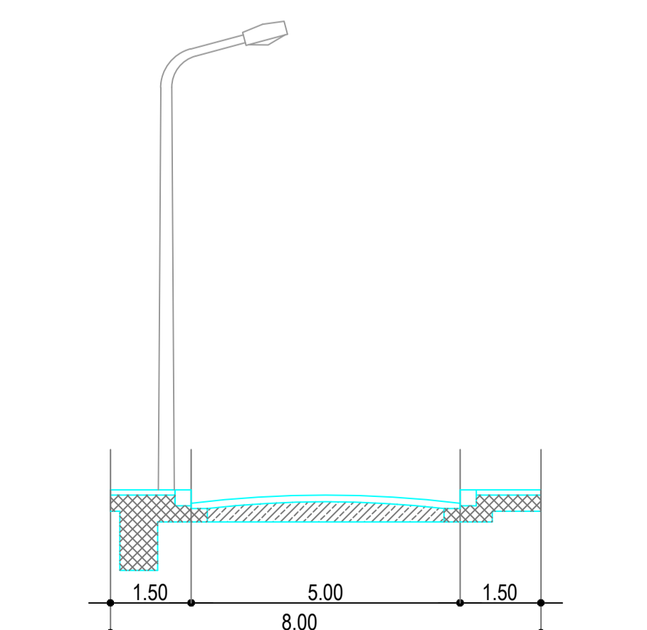
SEZ. D - D
