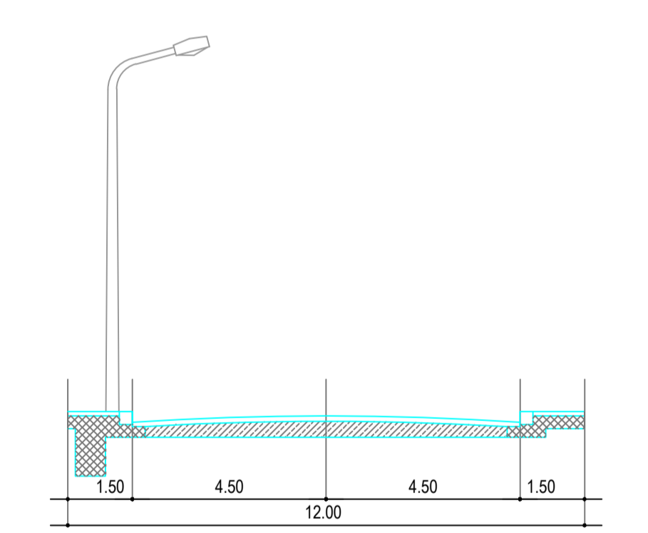
SEZ. B - B
