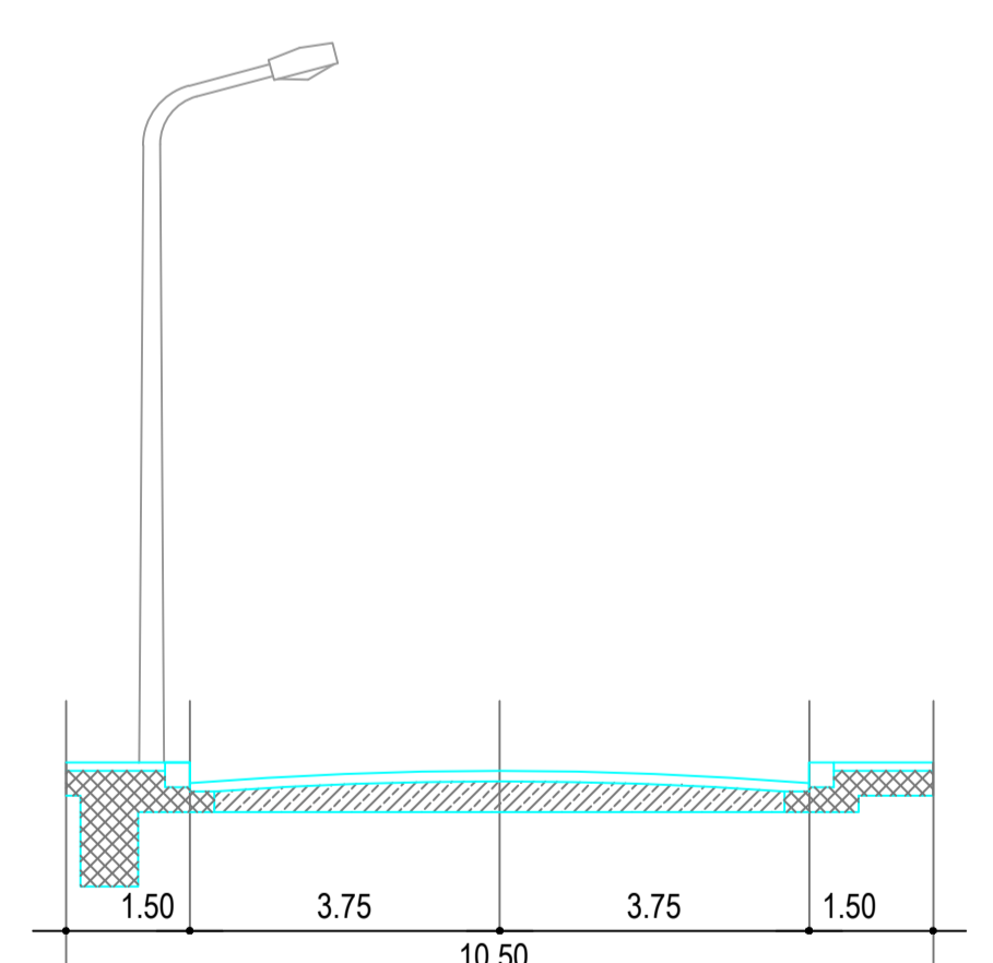
SEZ. C - C
