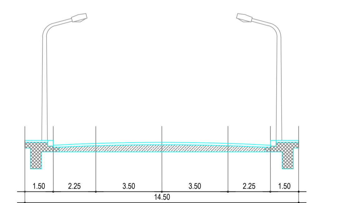
SEZ. A - A
