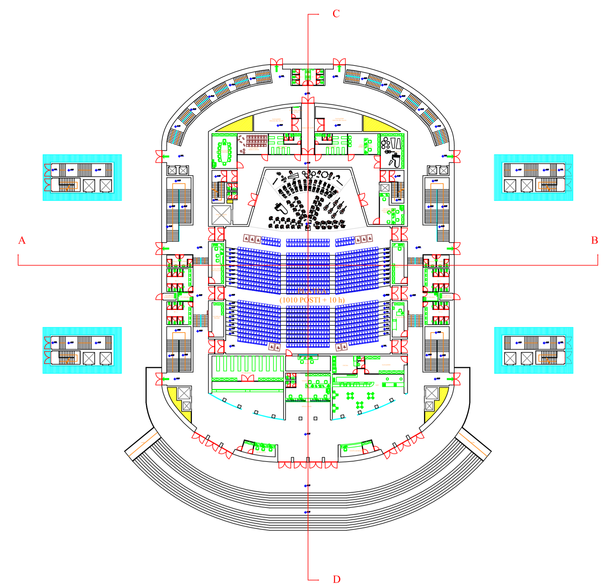
PLANIMETRIA PIANO TERRA (1010 posti + 10 h.)
